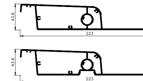
Lamela dachowa o wymiarach 44×223 mm
