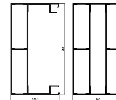
Platew skrajna i pośrednia o wymiarach 140×255 mm
